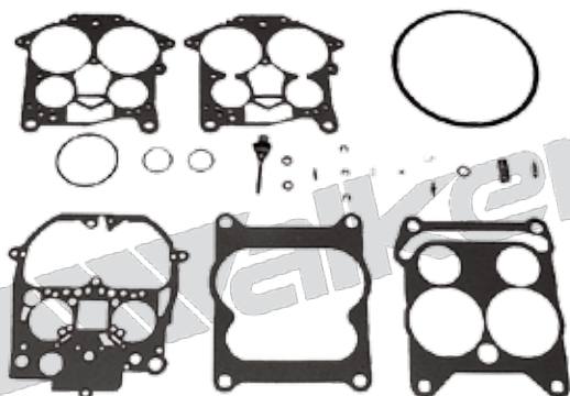
19033 (R-4) CRUSADER #45334 / MERCURUISER 823426A1, 1397-7539, 1397-7540, 1397-7544, 1397-8535, 1397-9723 OMC # 383918, 983864 / VOLVO # 834985-4
