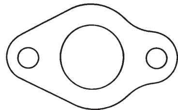
234F FLANGE GASKET
